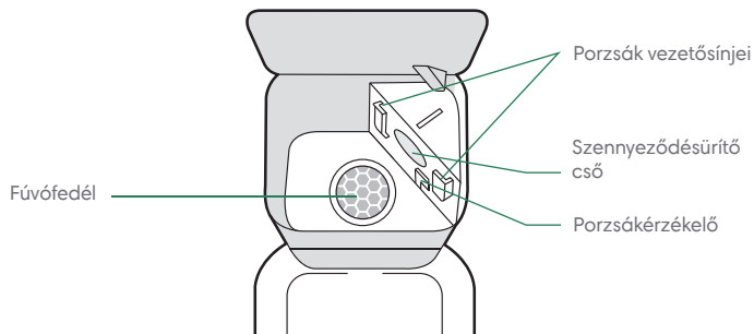
Felülnézet
